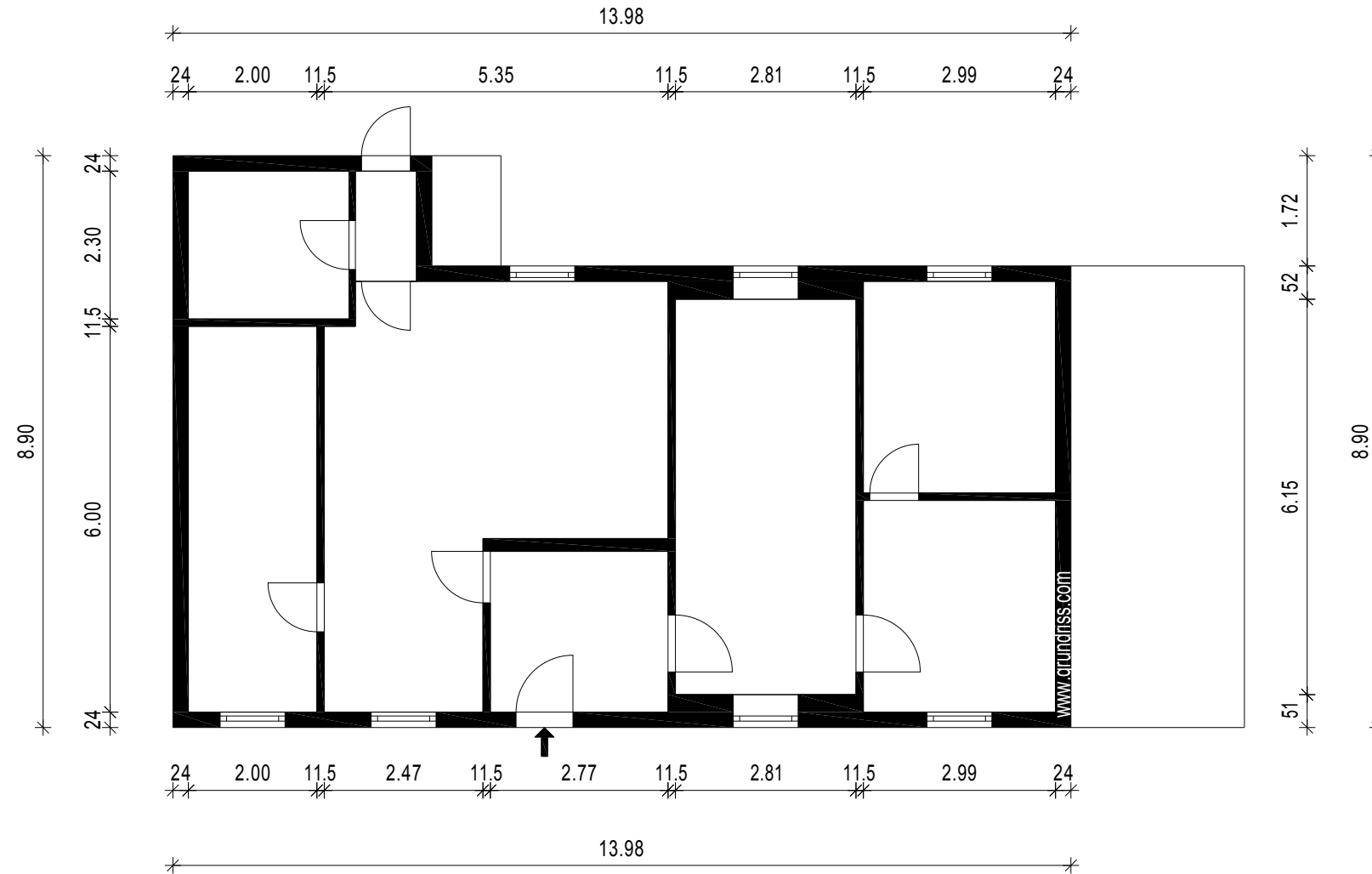
Grundriss Gabelsberger Straße 10 in Schöningen - Obergeschoss - Stand: 05/2021
