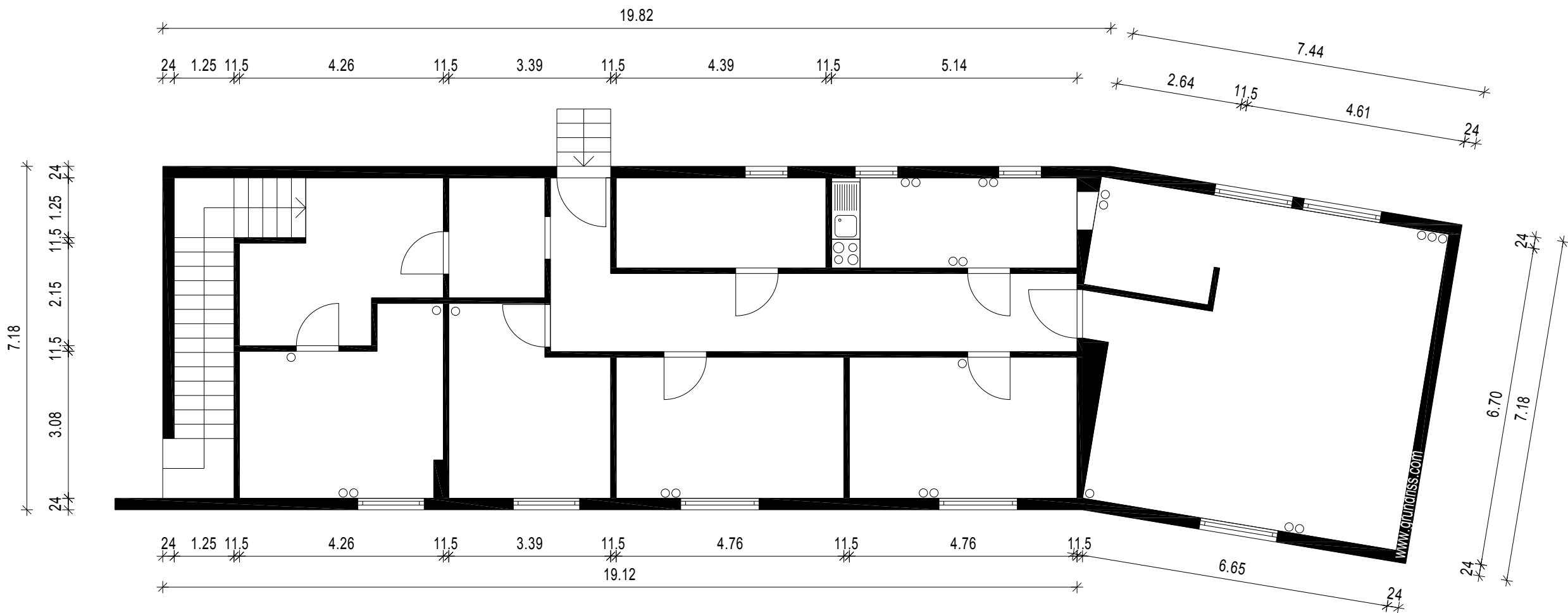
Grundriss Gabelsberger Straße 10 in Schöningen - Erdgeschoss - Stand: 05/ 2021
