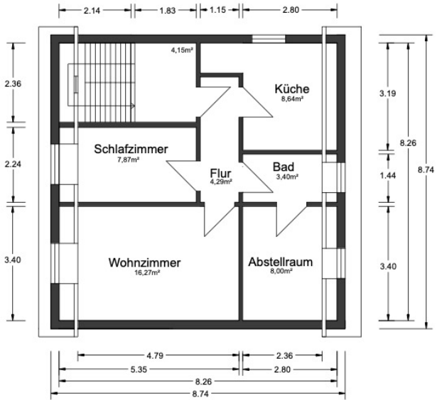
Grundriss EG
